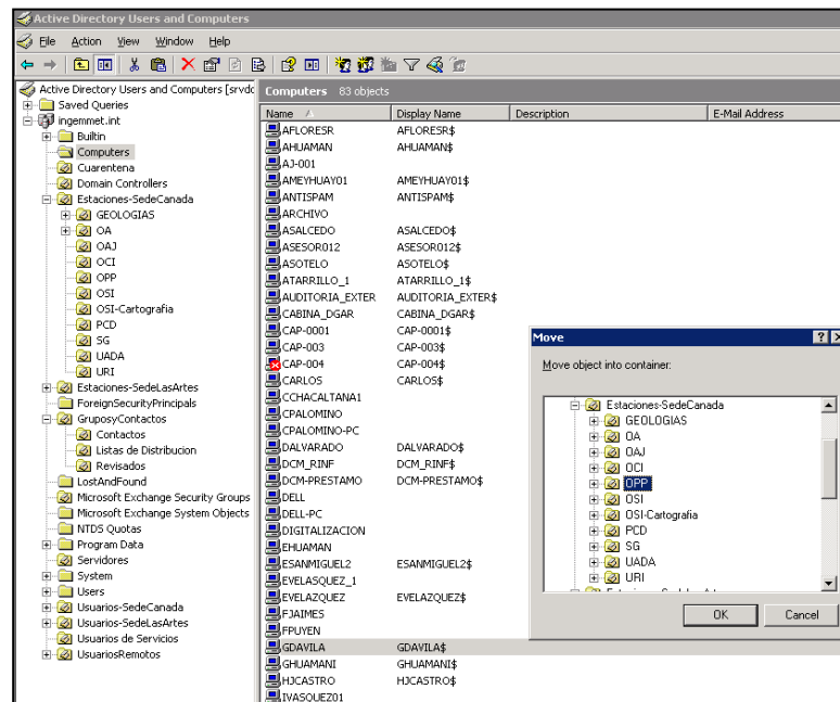
Fig. 03.- Ubicar el nombre del equipo en su respectiva área
